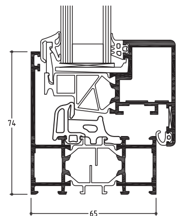
Coupe verticale
