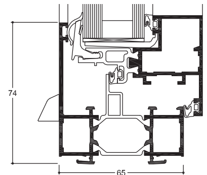
Coupe verticale
