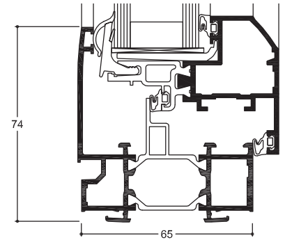
Coupe verticale
