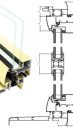
Coupe verticale
