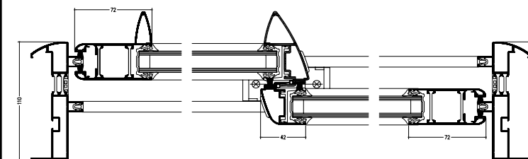
Coupe horizontale
