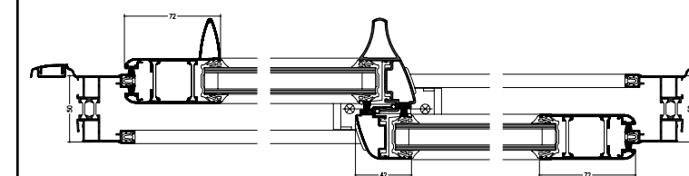
Coupe horizontale
