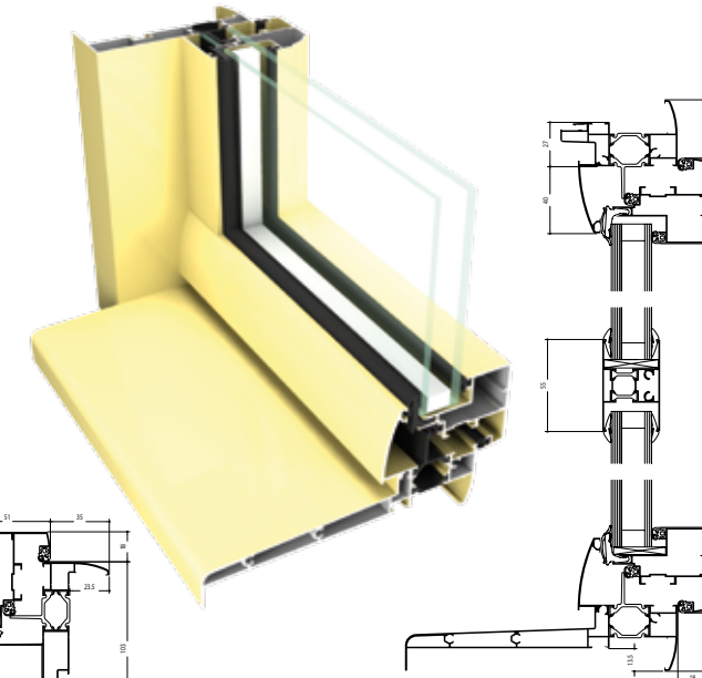
Coupe verticale
