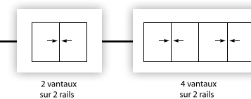
Coupe horizontale
