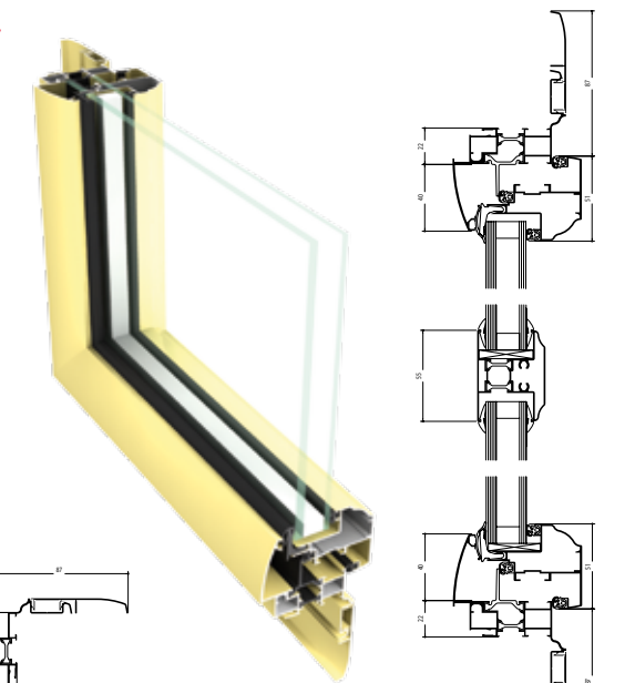
Coupe verticale
