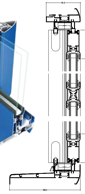
Coupe verticale
