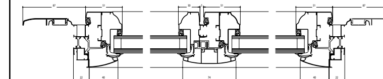
Coupe horizontale
