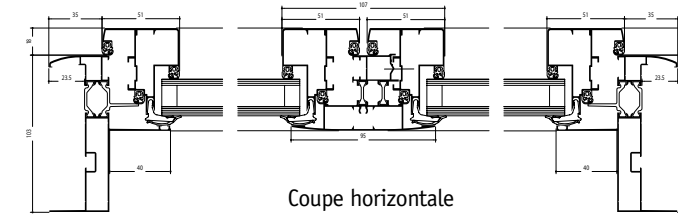
Coupe horizontale
