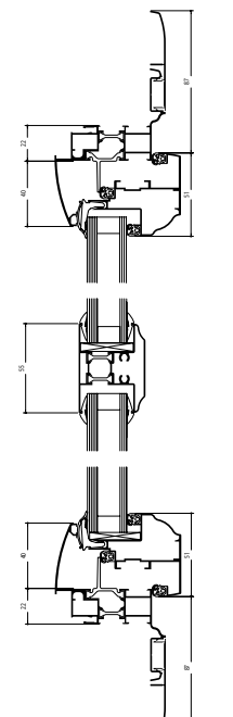
Coupe verticale
